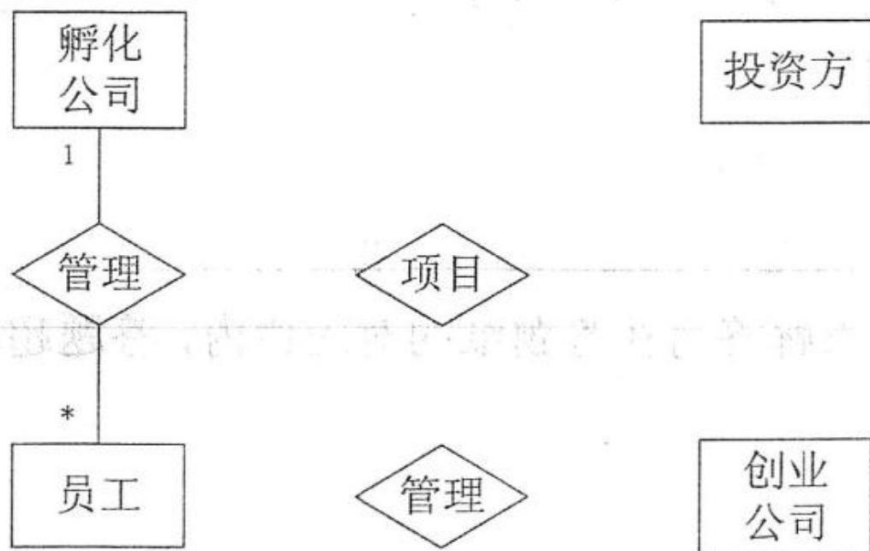
图 2-1 实体联系图
