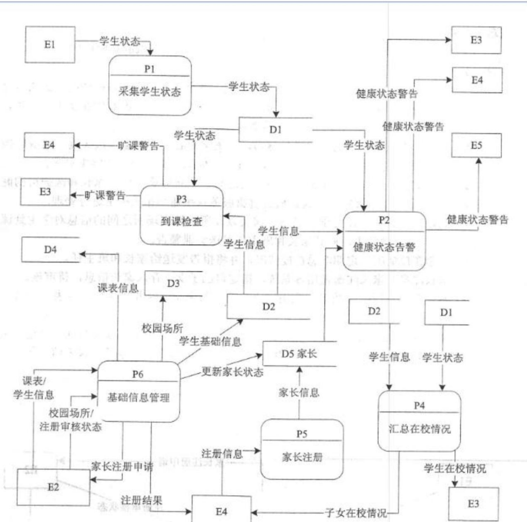
图 1-2 0层数据流图
