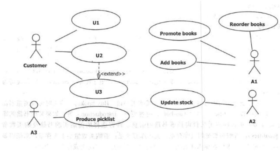
图 3-1 用例图
